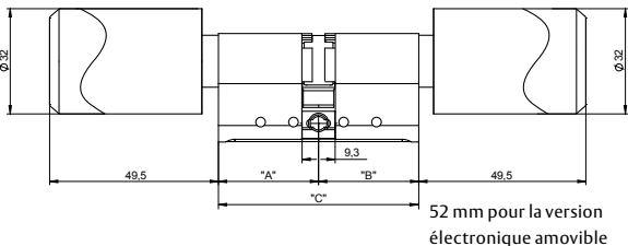
Dimensions du cylindre en mm
