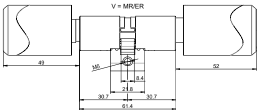
Dimensions du cylindre profil Suisse (en mm)
